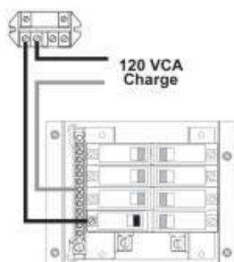
Relais de câblage pour équipement de piscine 120 VCA
