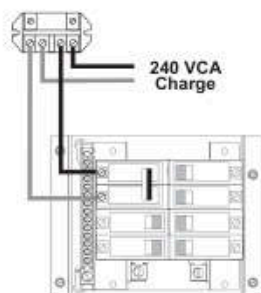
Relais de câblage pour équipement de piscine 240 VCA
