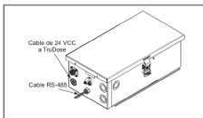
Figura 7. Conexión de comunicación/energía de TruClear XL
