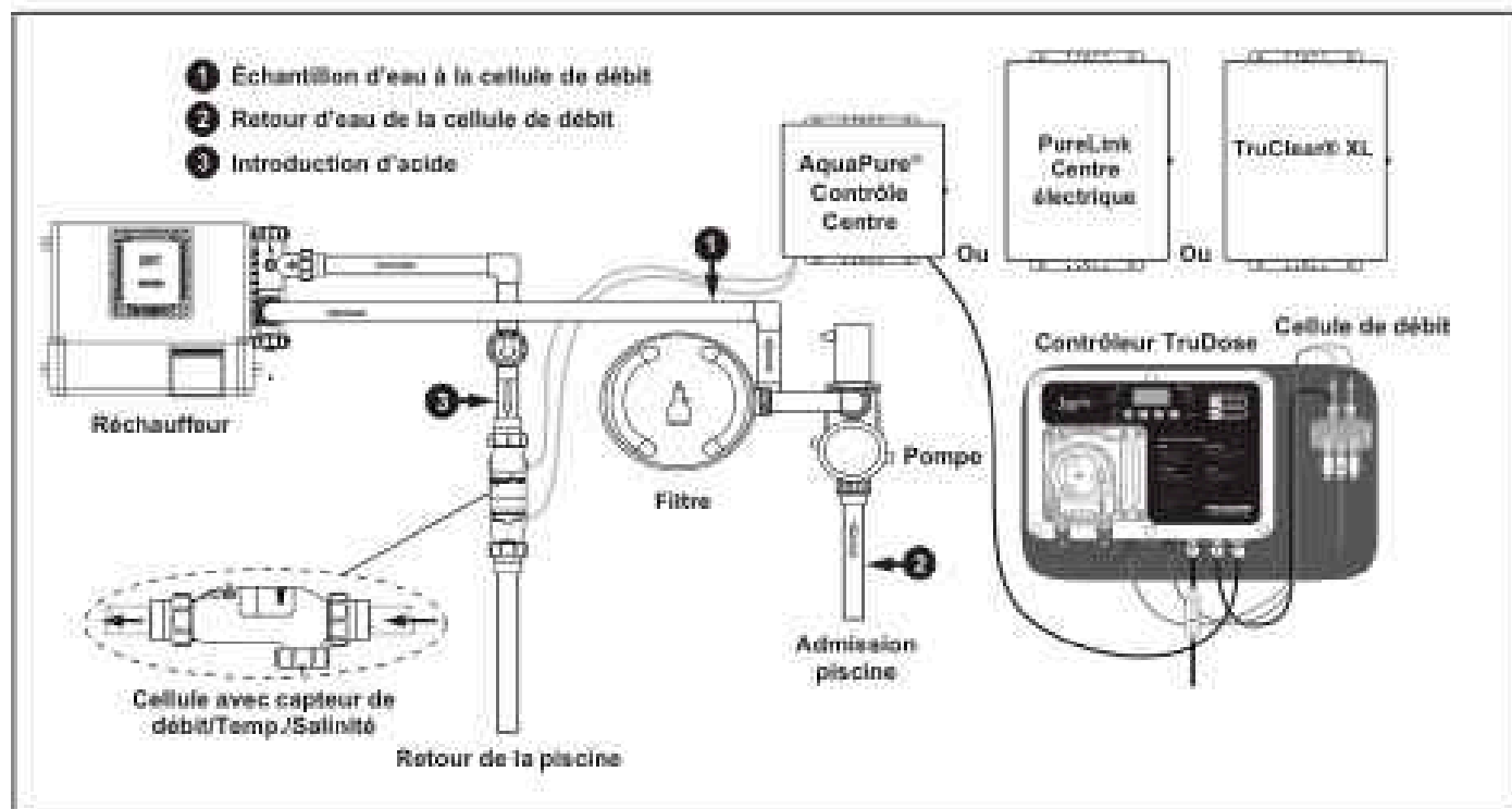
Figure 2. Connexion cellule de débit - Vue de haut
