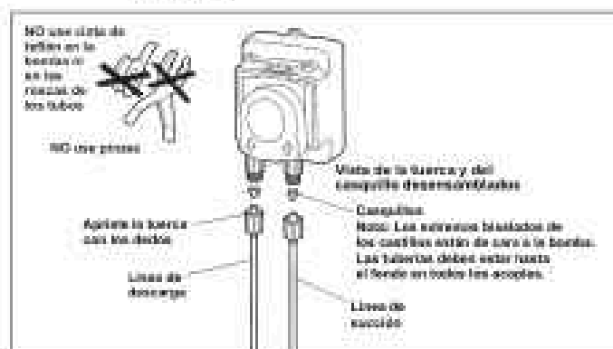
Figura 11. Instale la línea de succión al cabezal de la bomba
