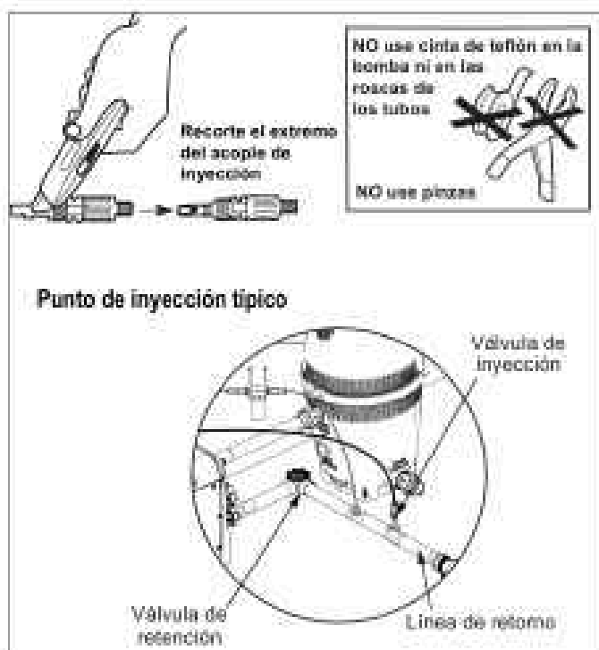
Figura 13. Instale la línea de descarga al cabezal de la bomba y al punto de inyección
