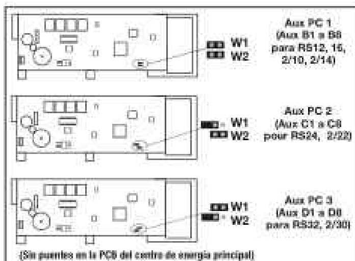
Figura 23. Configuración de los puentes para múltiples centros de energía auxiliar
