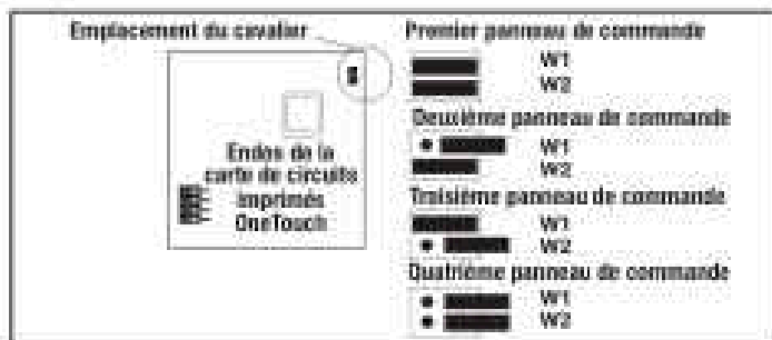
Figure 29. Réglages des cavaliers pour plusieurs panneaux de commande OneTouch™
