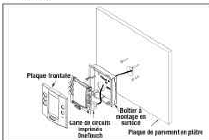
Figure 24. Montage en surface OneTouch™
