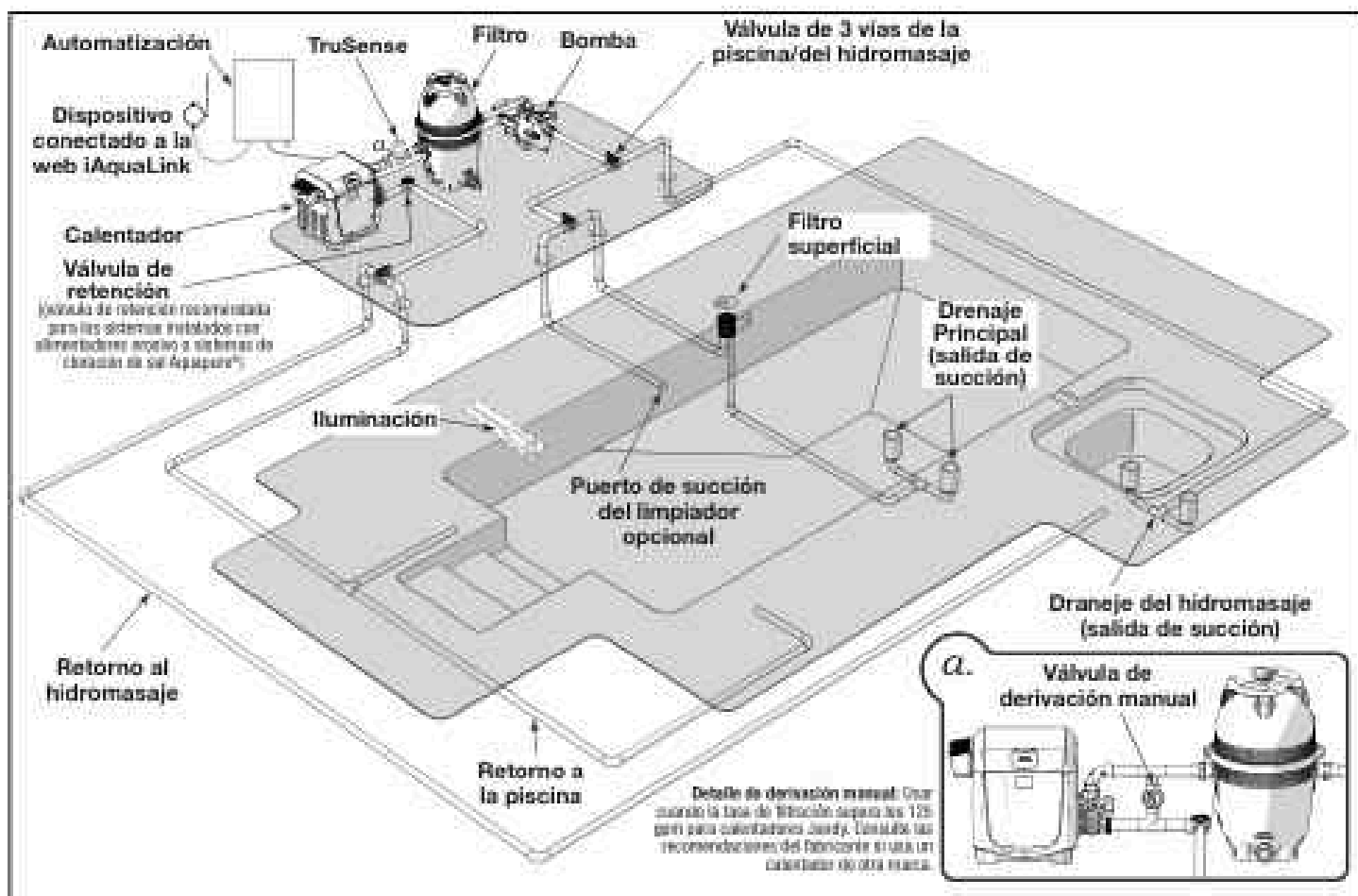
Figura 2. Configuración típica de las tuberías de agua
