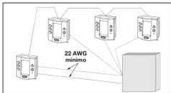
Figura 28. Instalación de múltiples paneles de control OneTouch
