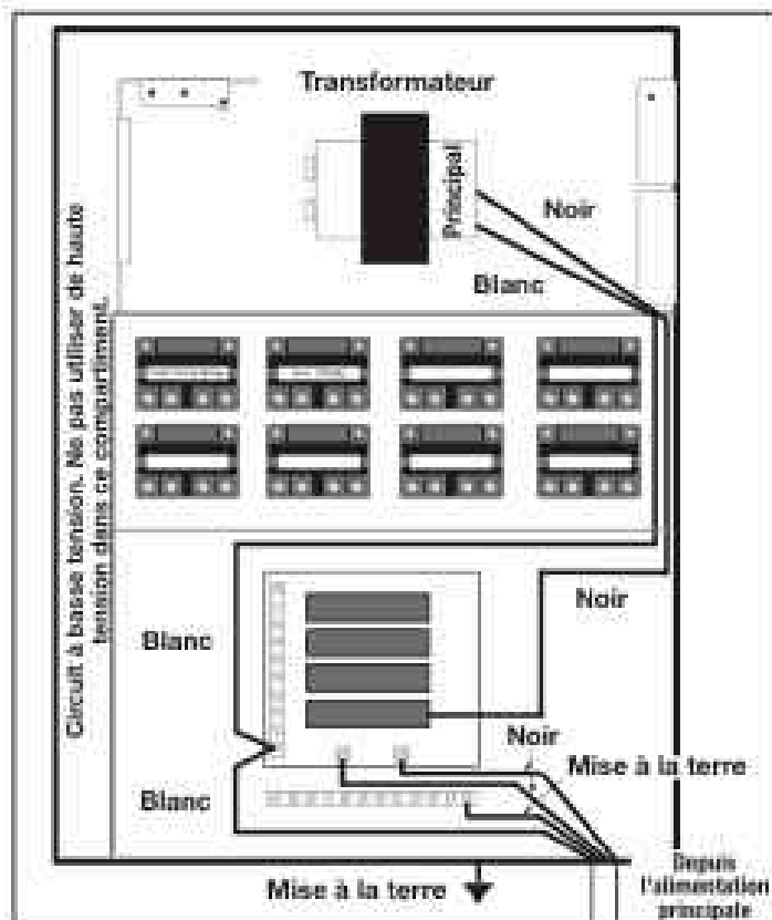
Figure 4. Centre électrique du sous-panneau
