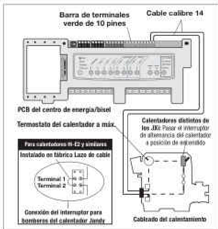
Figura 17. Conexión del calentador de Jandy
