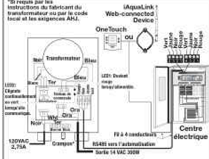
Figure 9. Câblage des lumières DEL au contrôleur pour lumière DEL Infinite WaterColors
