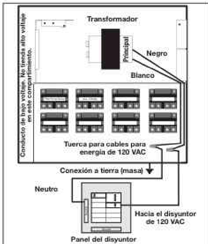
Figura 3. Centro de energía estándar
