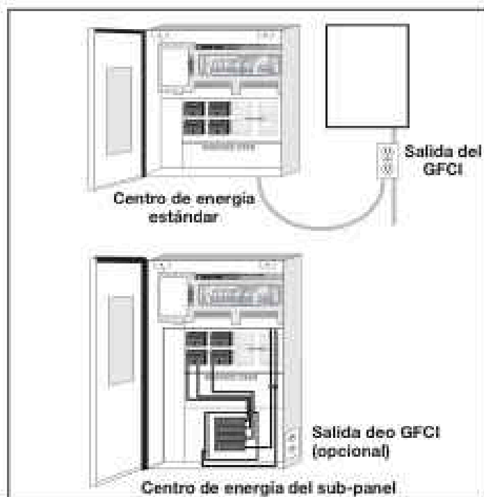
Figura 6. Instalación del GFCI para la iluminación sumergida de alto voltaje
