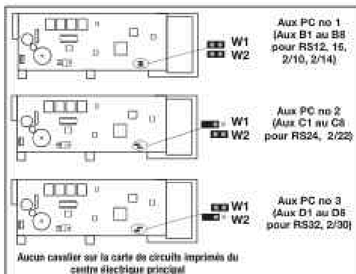
Figure 23. Mise en place des cavaliers pour plusieurs centres électriques auxiliaires
