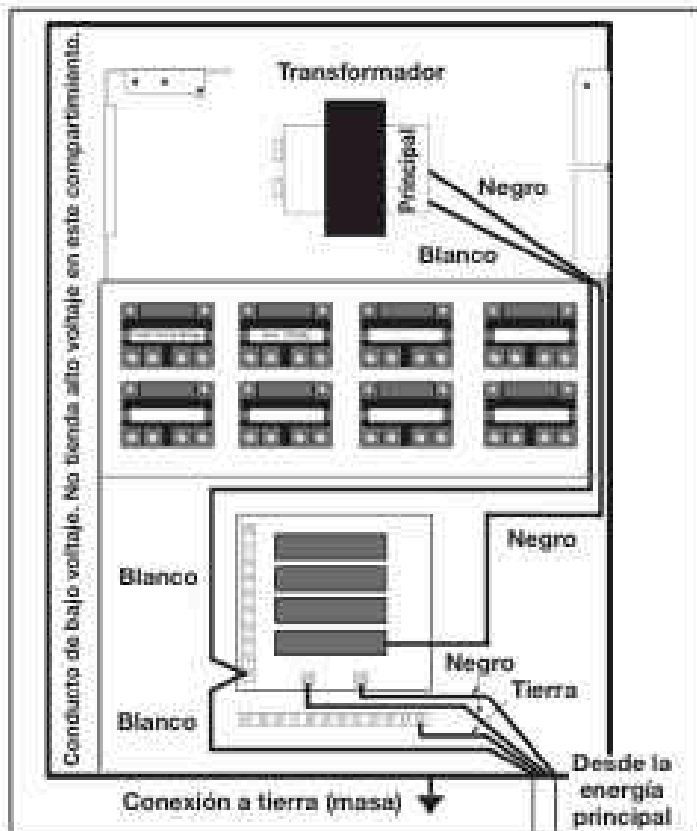
Figura 4. Centro de energía del subpanel
