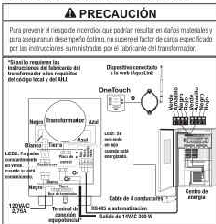
Figura 9. Cableado de las luces LED al controlador de luces LED Infinite WaterColors
