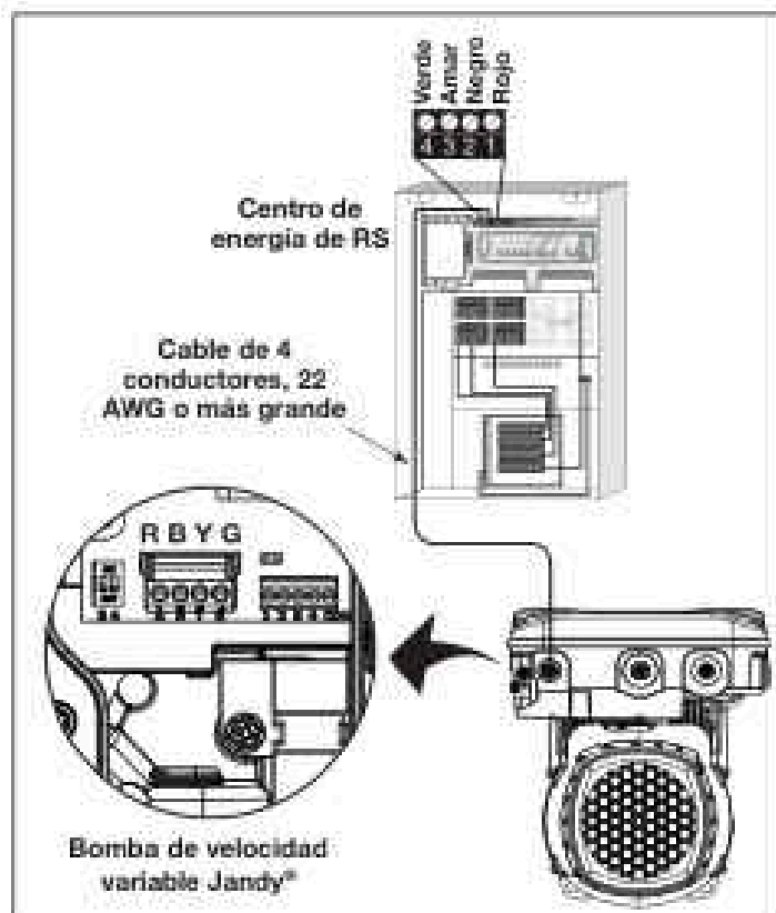
Figura 14. Cableado de bajo voltaje para la bomba de velocidad variable Jandy
