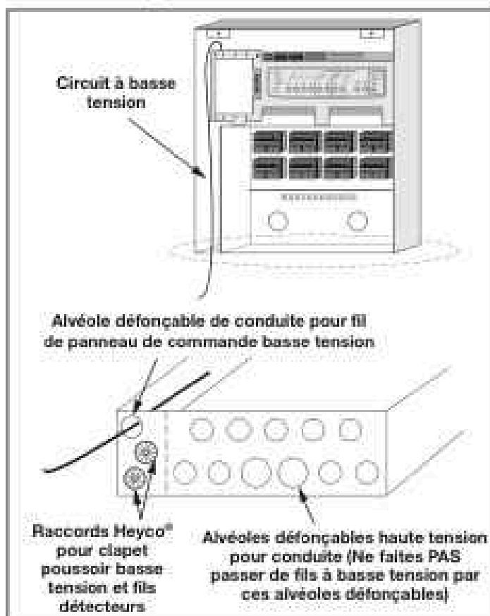
Figure 13. Câble du panneau de commande à la carte de circuits imprimés du centre électrique
