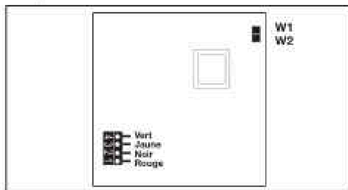
Figure 25. Vue arrière - Carte de circuits imprimés OneTouch
