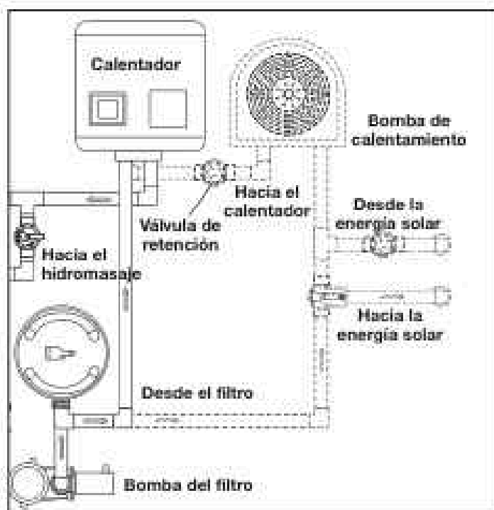
Figura 1. Tuberías de la bomba de calentamiento.
