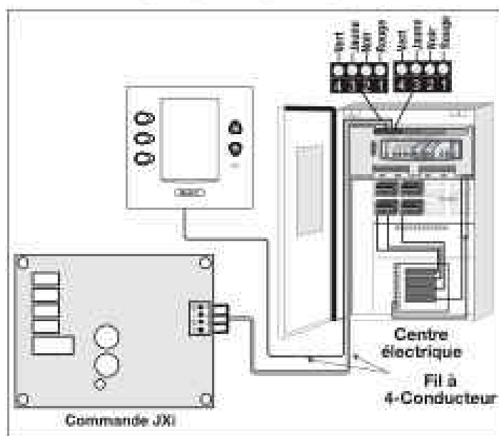
Figure 18. Connexion de l'appareil de chauffage JXi de Jandy au centre électrique
