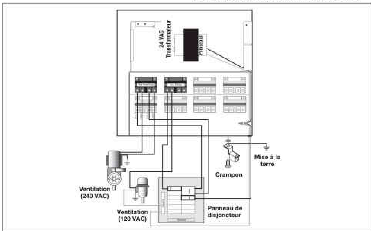
Figure 5. Centre électrique standard - Métallisation
