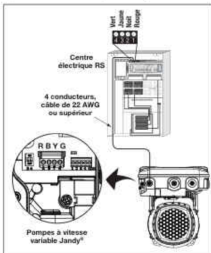
Figure 14. Câblage à basse tension pour la pompe à vitesse variable Jandy
