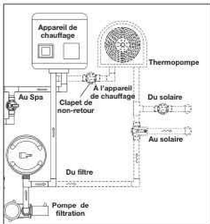
Figure 1. Plomberie pour thermopompe
