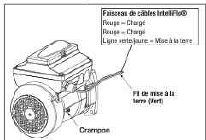
Figure 11. Mise à la masse externe Pentair
