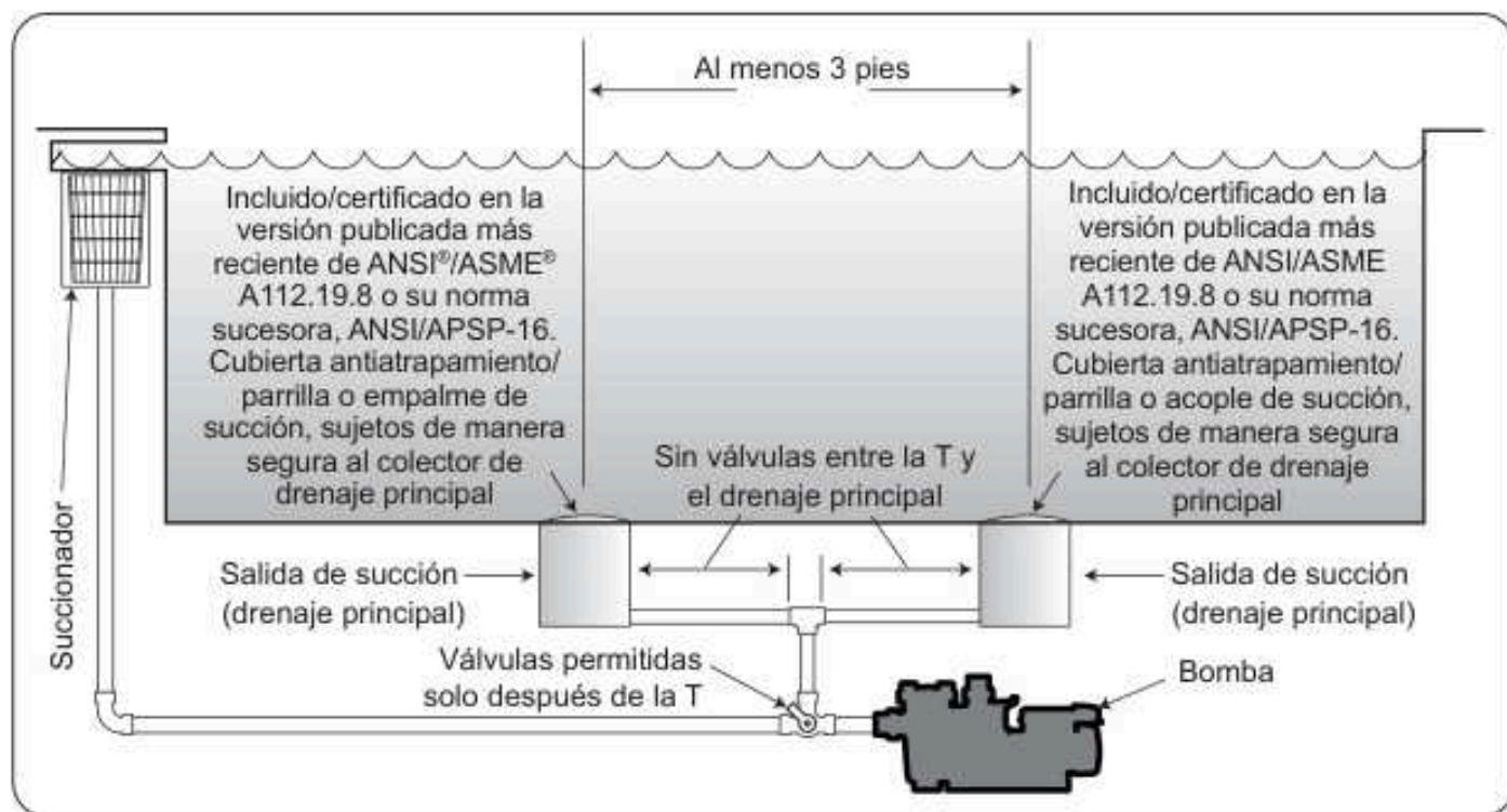
Figura 1. Cantidad de salidas de succión por bomba
