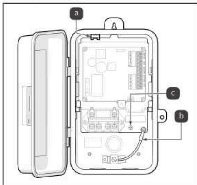
Figura 11. Montaje y conexión a tierra del chasis de TCX
