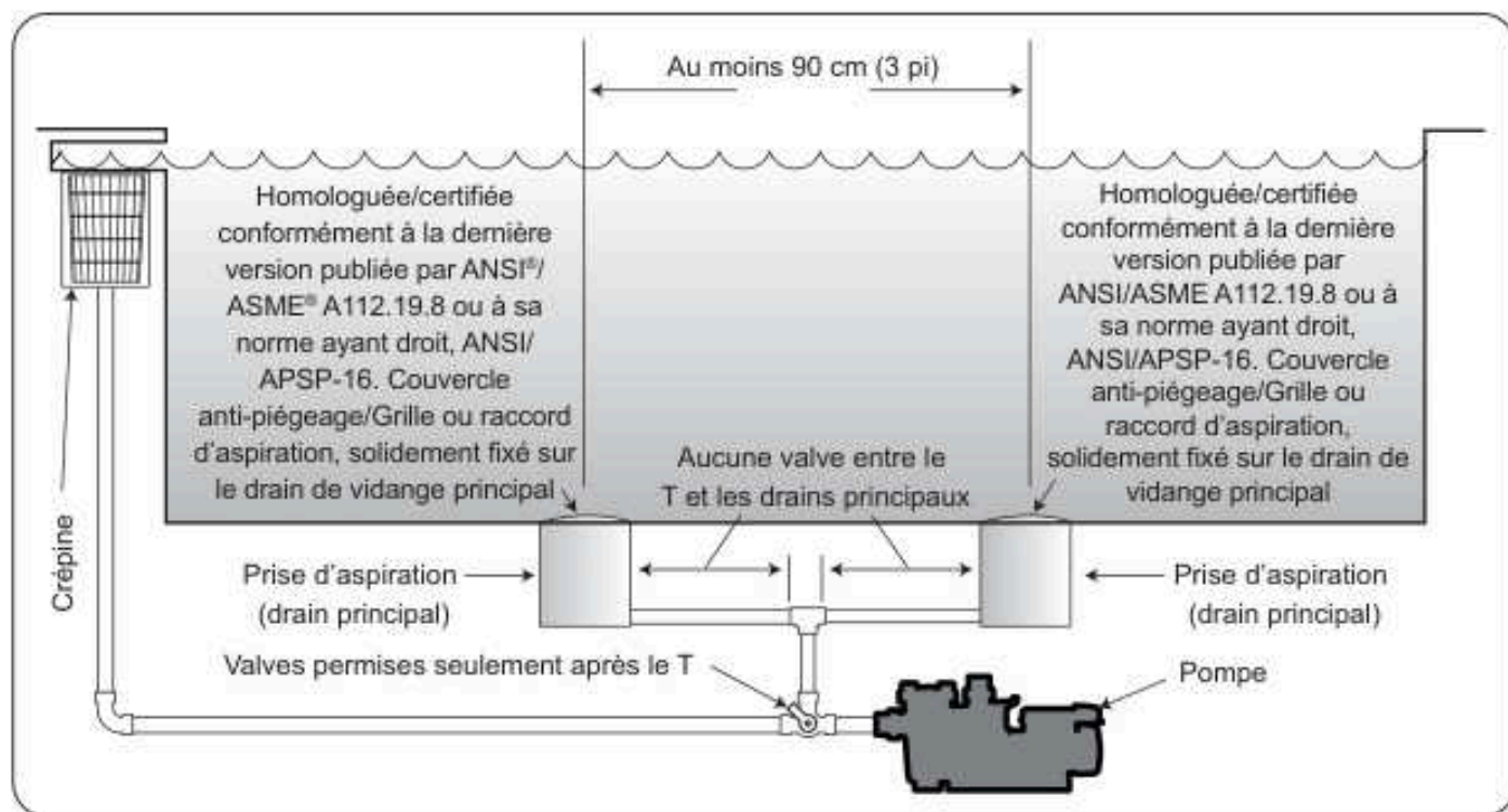
Figure 1. Nombre de prises d'aspiration par pompe
