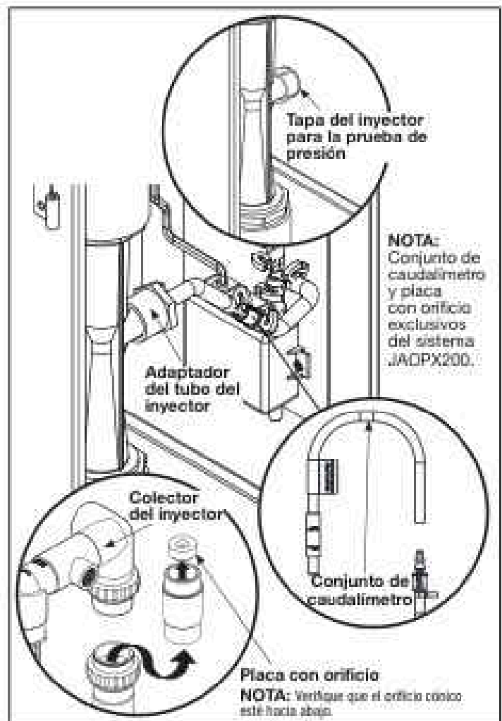
Figura 6. Pruebas de flujo y presión del sistema AOP Jandy
