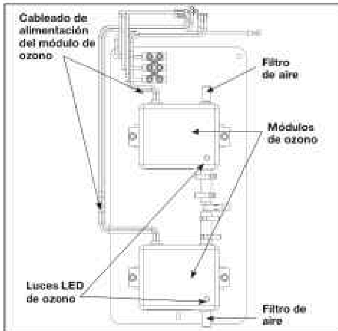
Figura 11. Vista ortográfica general del sistema generador de ozono
