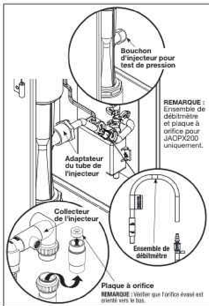
Figure 6. Test de débit et de pression Jandy AOP
