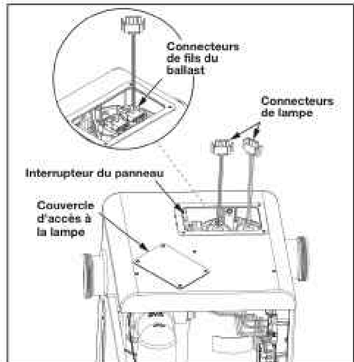
Figure 21. Accès à la lampe du réacteur UV du système Jandy AOP
