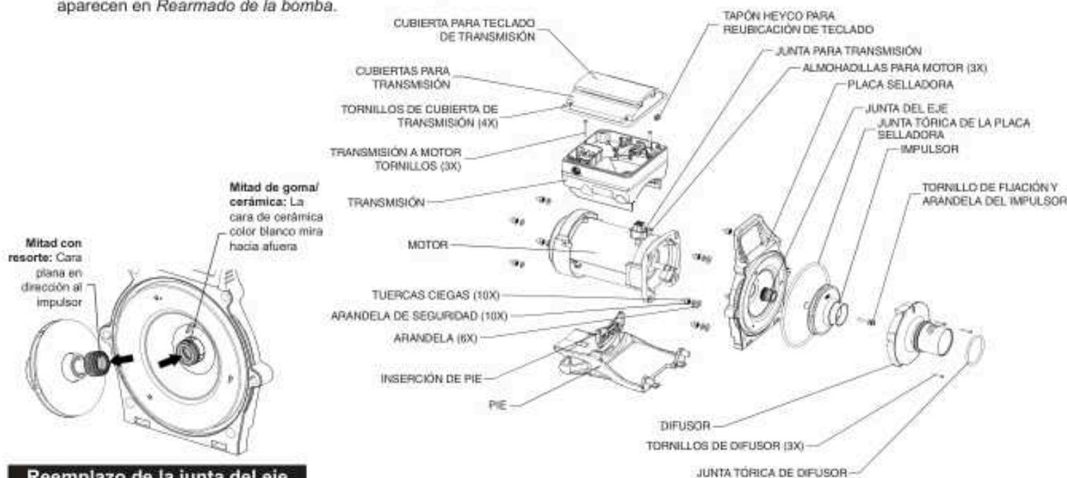
Detalles del ensamblaje del motor
