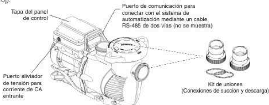
Ensamblaje de transmisión de velocidad y flujo variable
