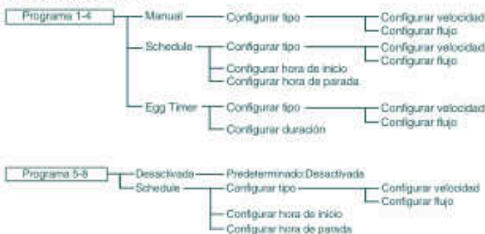
Opciones del árbol del menú de programas
