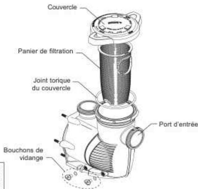
Ensemble du boîtier de la crépine
