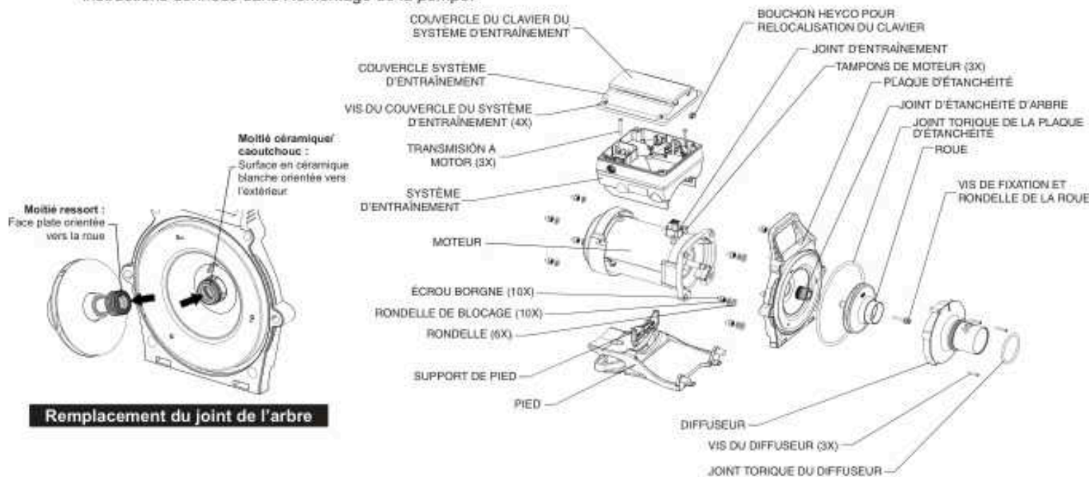
Analyse de l'ensemble moteur
