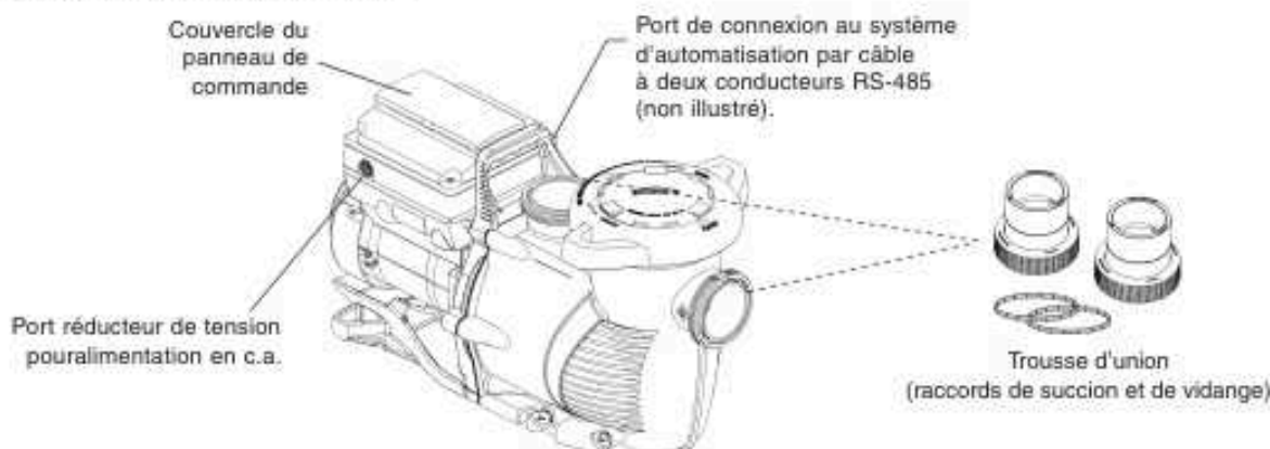
Ensemble du système d'entraînement à vitesse et débit variable
