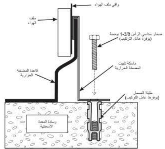
تركيب قامطة (قامطات) التثبيت
