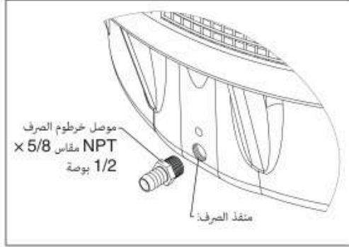
تركيب موصل خرطوم الصرف
