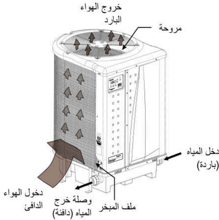
دورة التسخين النموذجية
