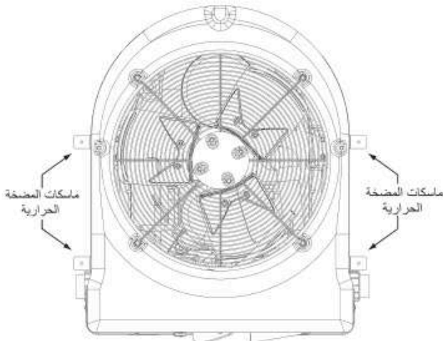
تركيب قامطة (قامطات) التثبيت
