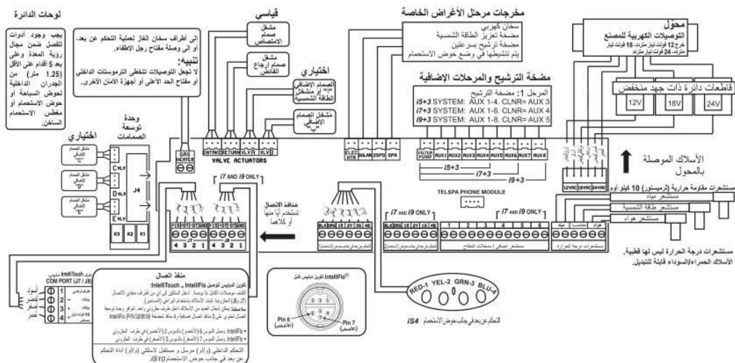
مخطط أسلاك مركز التحميل IntelliTouch/EasyTouch
