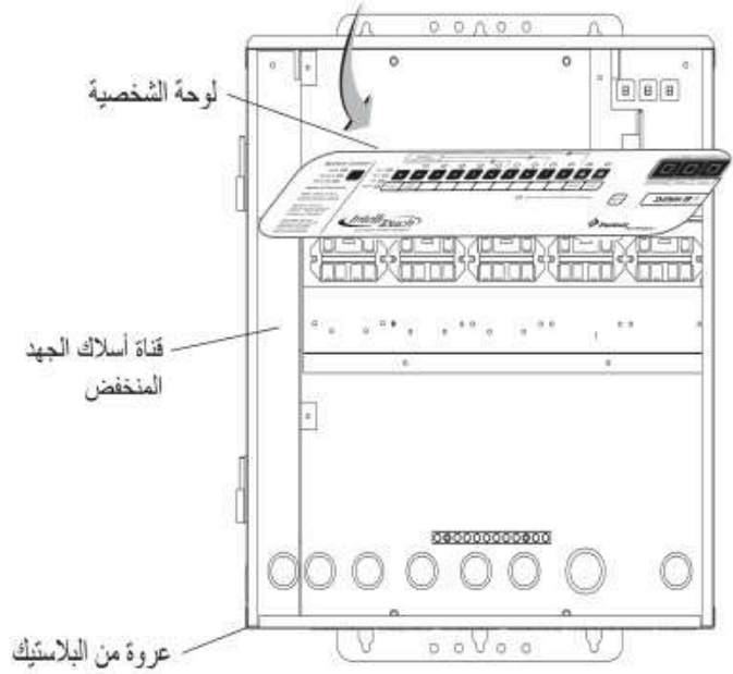
مركز حمل IntelliTouch
