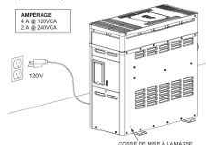
Figure 17. Alimentation de l'appareil
