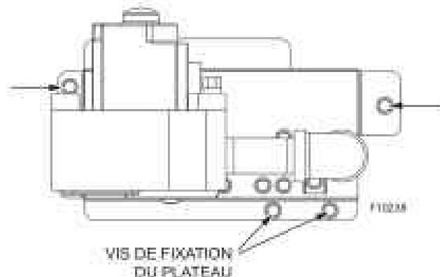
Figure 41. Retrait de la vanne de gaz
