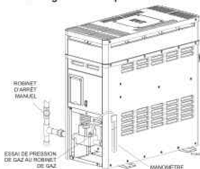
Figure 11. Réglage de la pression du gaz
